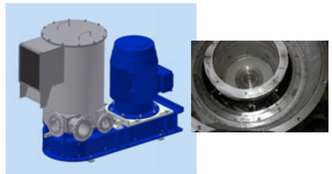
Třídíč CRS (optimalizace dotřídění výplivů) / CRS screen (optimization of rejects final screening)
