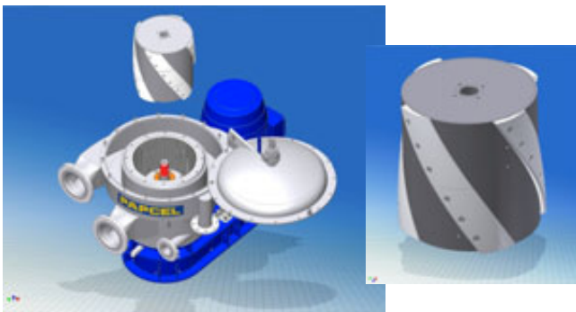
STU ve stupni hrubého třídění, nový typ lopatkového rotoru EHD pro hrubé třídění / STU in the stage of coarse screening, new type of vaned rotor EHD for coarse screening
