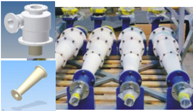
Plastové kužele vířivých třídíčů / Plastic cones of vibrating cleaners
